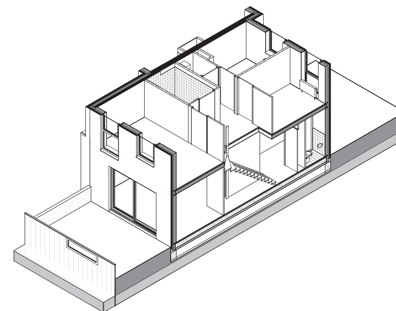
3D eerste verdieping
