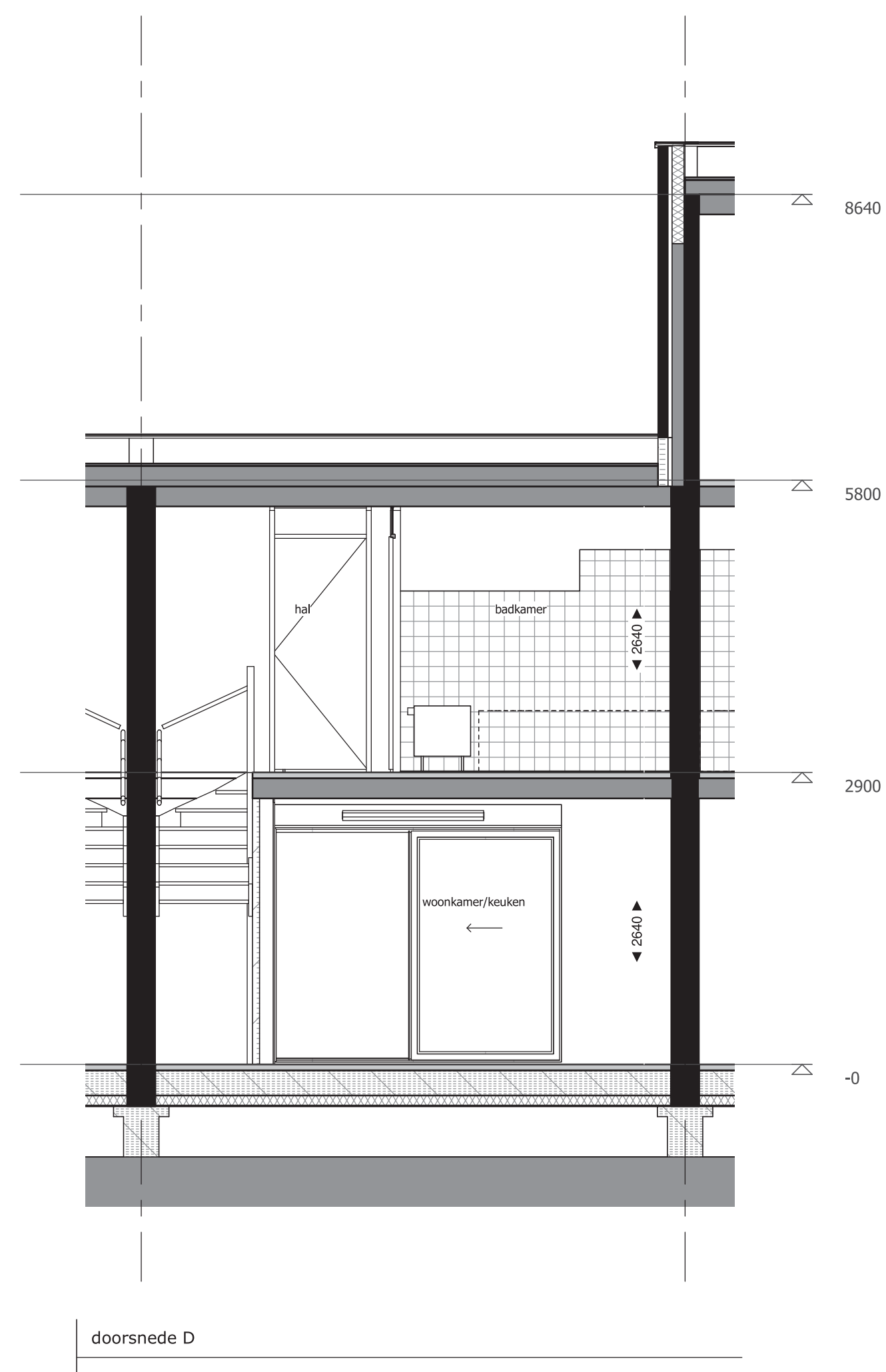
doorsnede D 1:50
